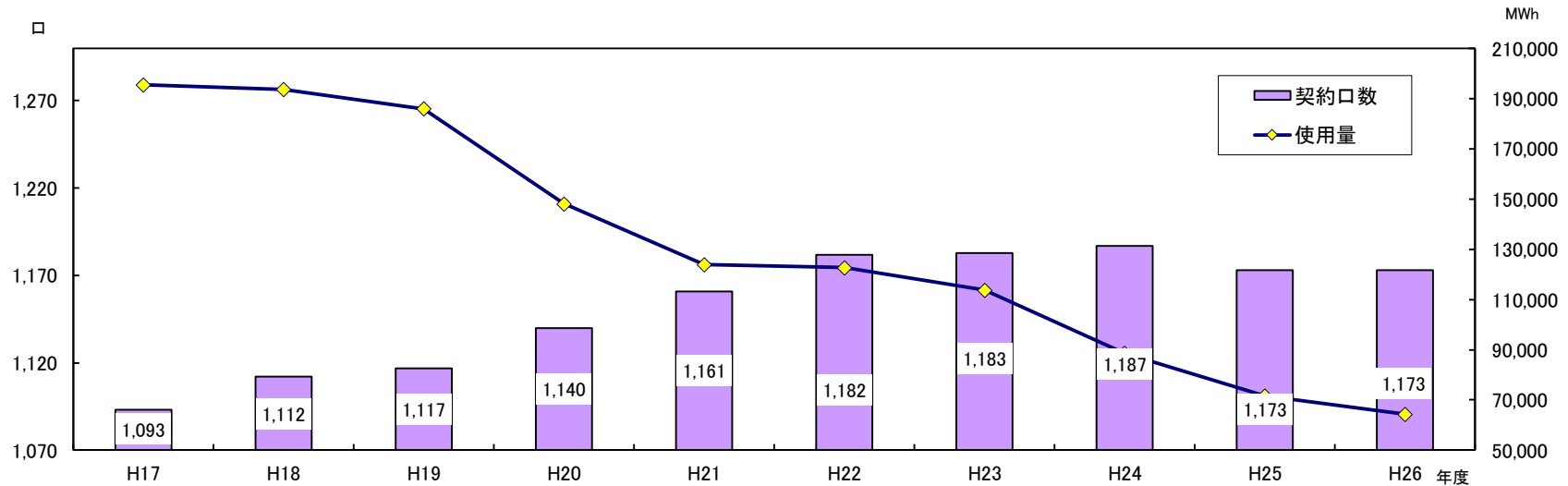
年度別電力契約口数及び使用量の推移
